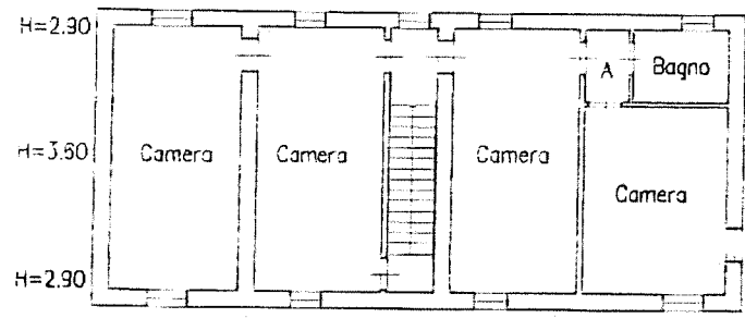
PIANO PRIMO
