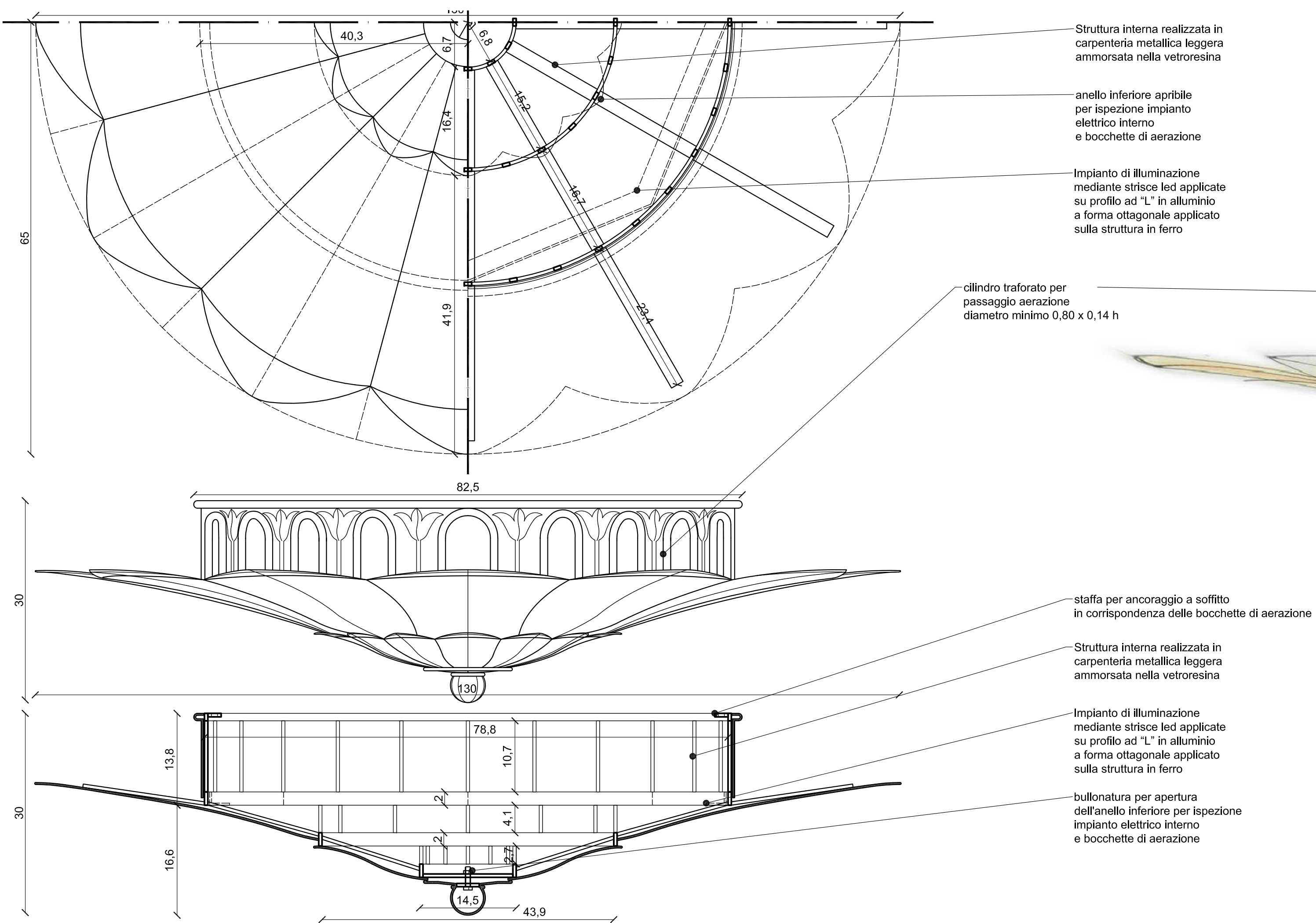
LAMPADARIO SALA "A" - scala 1:5
